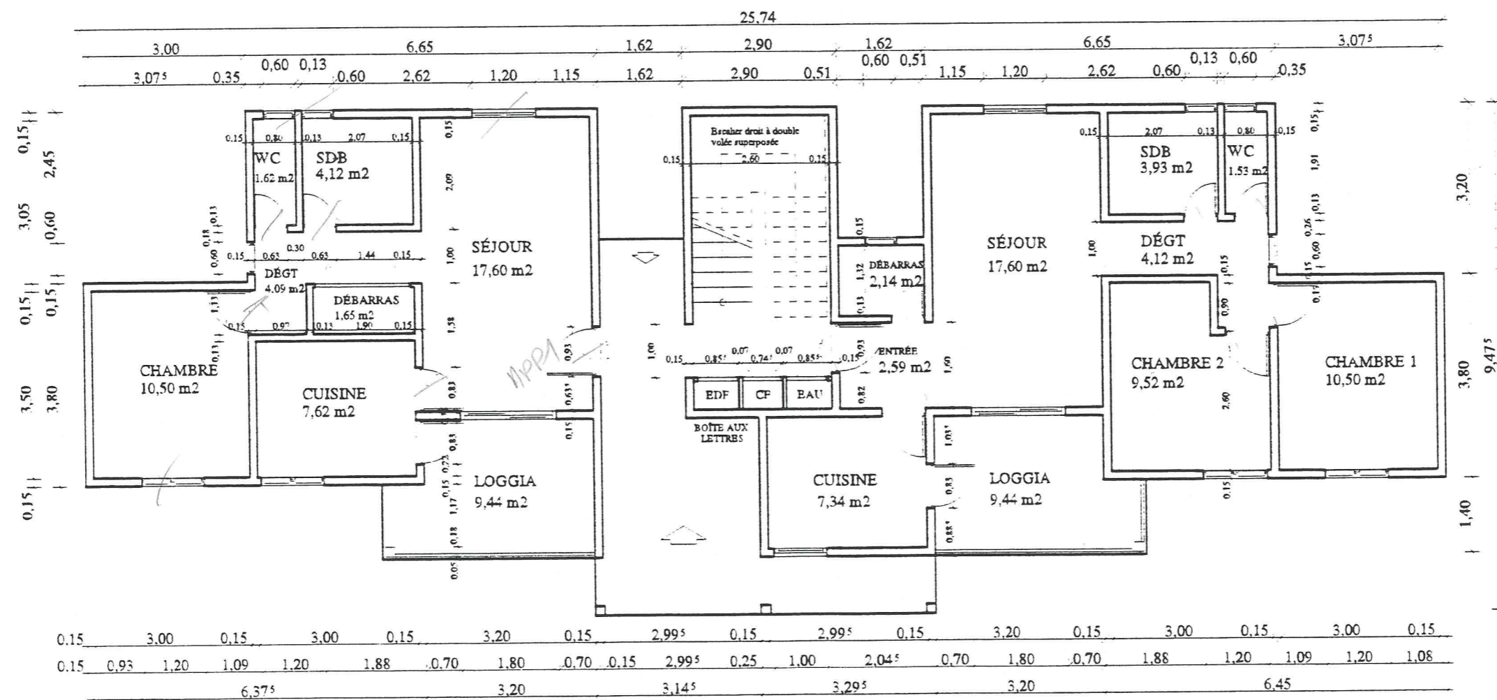
PLAN DU REZ DE CHAUSSEE Bât 1, 2, 9 & 10
